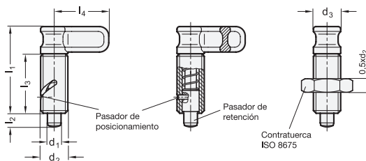
Pasador de retención retraído
