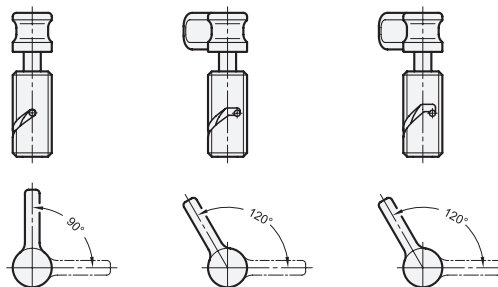
Pasador de retención retraído
